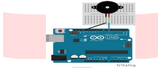
Gambar 4 Arduino dan Buzzer [16]
