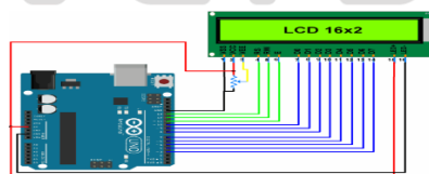
Gambar 3 Arduino dan LCD [3]
