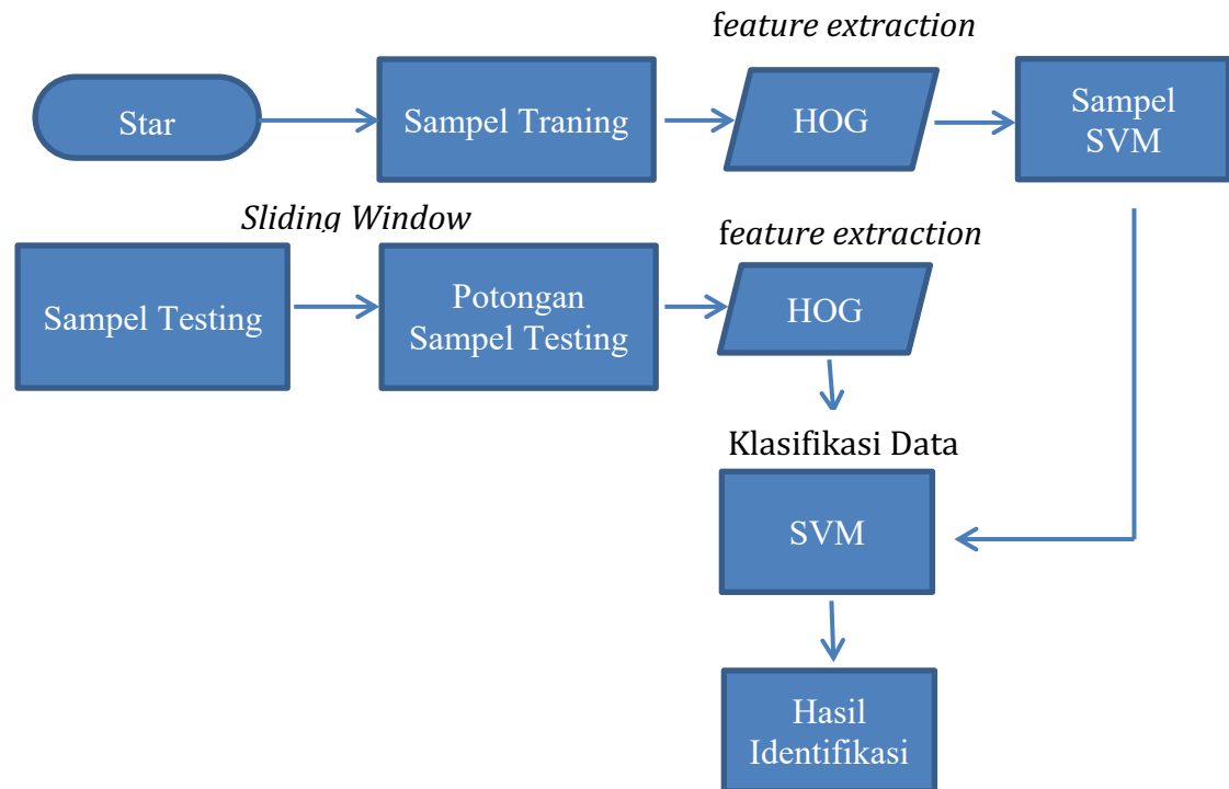
Gambar 3.1 Alur Sistem
