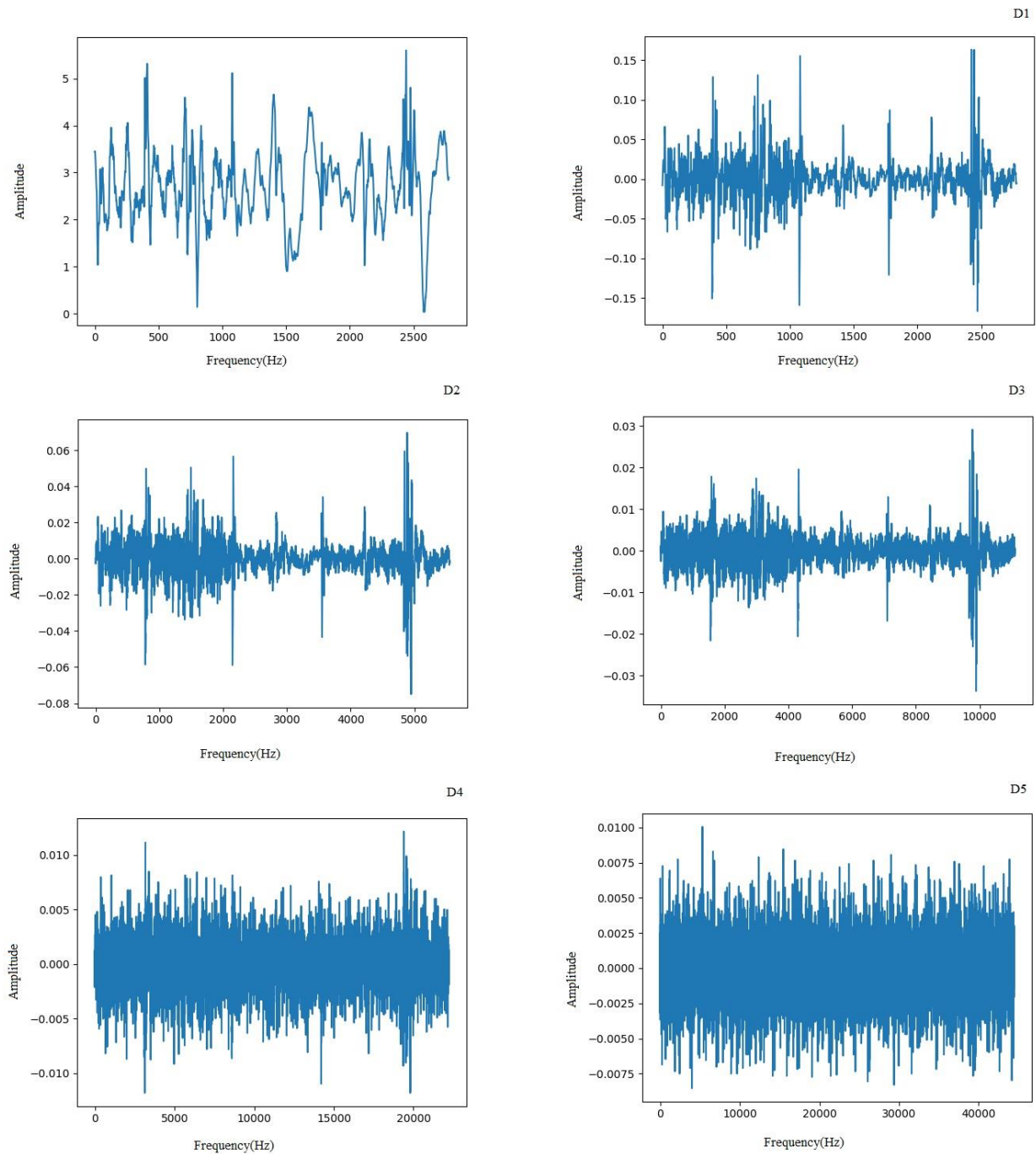
Gambar 2. Dekomposisi wavelet
