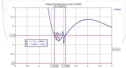
Gambar 3. Hasil Simulasi Antena VSWR
