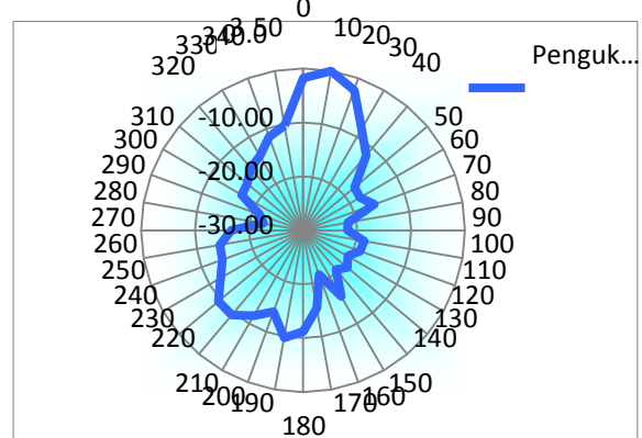
Gambar 15. Hasil Pengukuran Polaradiasi Elevasi
