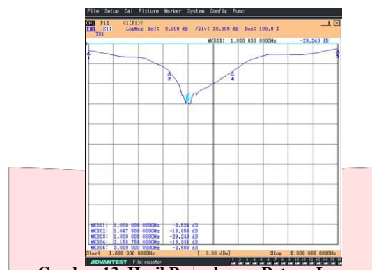
Gambar 13. Hasil Pengukuran Return Loss
