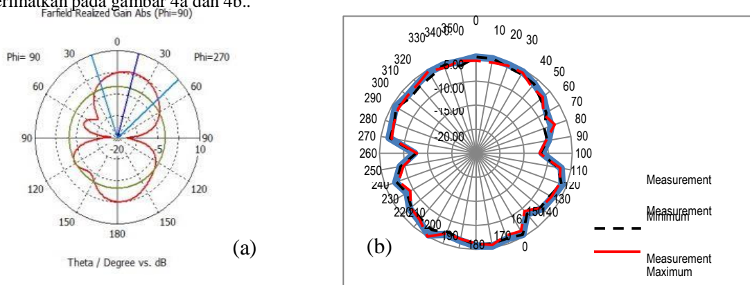
Gambar 4(a),(b) : Pola Radiasi Elevasi Antena Cloverleaf
