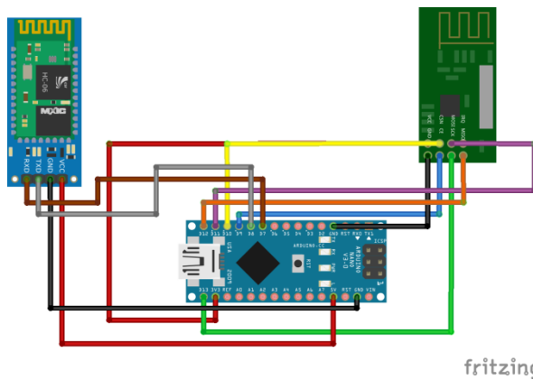
Gambar 2.8 : desain rangkaian pada kordinator
