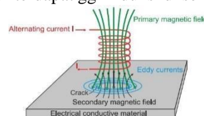
Gambar 2.3 Arus Eddy yang dihasilkan medan magnetik melalui objek[1].
