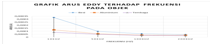
Gambar 4.6 Grafik Arus Eddy yang terjadi pada Objek
