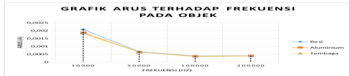
Gambar 4.5 Grafik Arus pada Koil Samping-Samping
