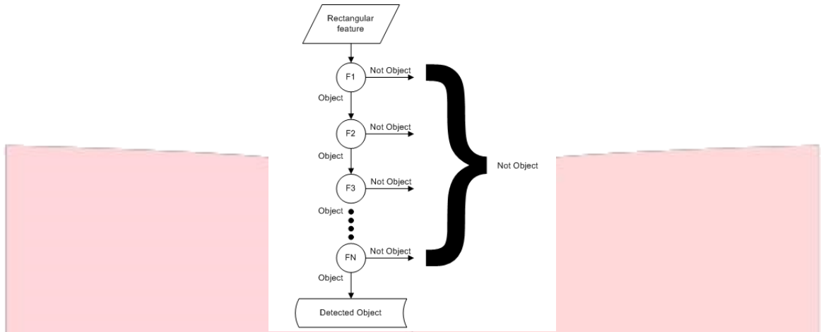
Gambar 2.4 Cascade Clasifier
