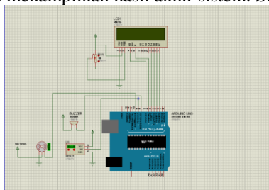
Gambar 3.4 Skema Rangkaian
