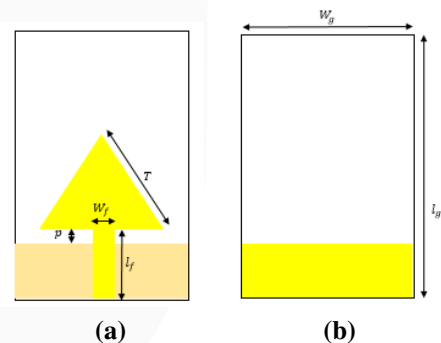
GAMBAR 1 (Desain Rancangan Awal, (a) Tampak Depan, (b) Tampak Belakang)
