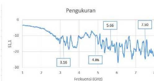
GAMBAR 2 (Hasil Return Loss Pengukuran)
