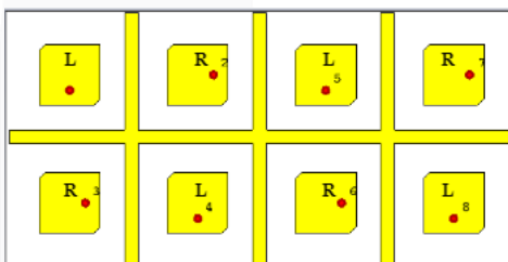
GAMBAR XII ANTENA DELAPAN ELEMEN KONFIGURASI 2 MENGGUNAKAN ISOLATION WALL
