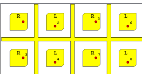
GAMBAR XIII ANTENA DELAPAN ELEMEN KONFIGURASI 3 MENGGUNAKAN ISOLATION WALL
