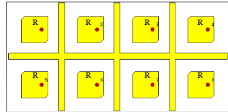
GAMBAR IX ANTENA DELAPAN ELEMEN KONFIGURASI 1 MENGGUNAKAN ISOLATION WALL
