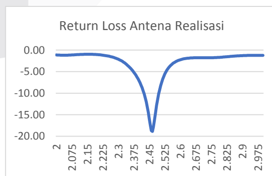
GAMBAR 4. 5 (Grafik Return Loss Antena Realisasi Tanpa Objek.)
