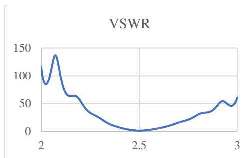
GAMBAR 4. 2 (Grafik VSWR Antena Simulasi Tanpa Objek.)
