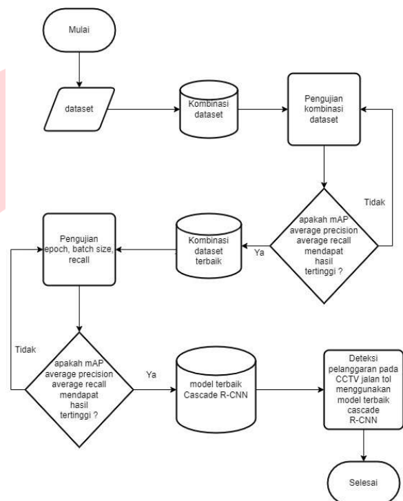
Gambar 15. Flowchart pembuatan model terbaik
