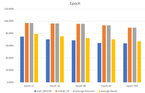
Gambar 10 Grafik pengujian epoch
