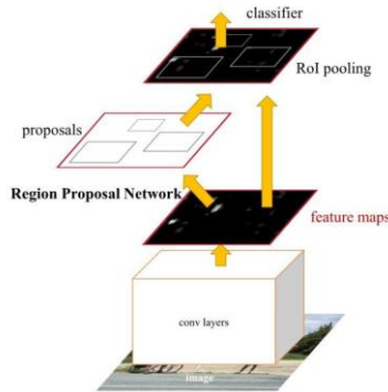
Gambar 5. Arsitektur Faster R-CNN [10]
