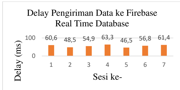
GAMBAR 12 Hasil Pengujian Delay
