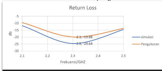
Gambar 4. 1 S-Parameter hasil simulasi dan pengukuran
