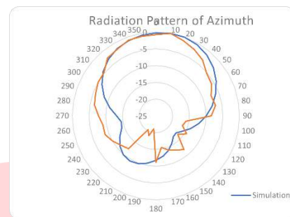
Gambar 4. 2 Pola Radiasi Azimuth
