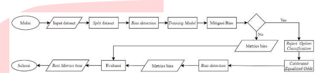
GAMBAR 4 Flowchart post-processing pada mitigasi bias
