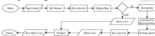
GAMBAR 2 Flowchart Pre-Processing pada mitigasi bias
