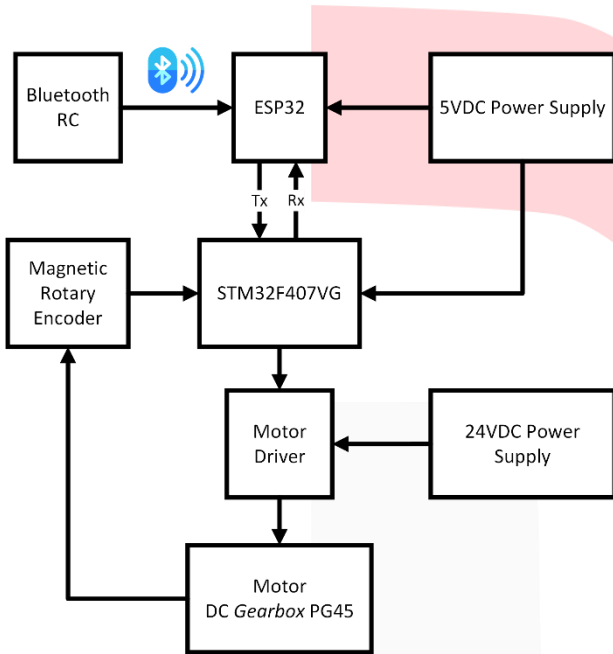
GAMBAR 8. Skematik elektronika sistem (B)
