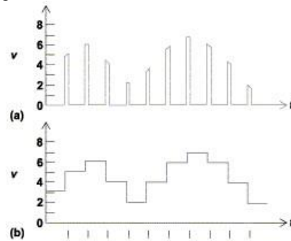
Gambar 3. Proses kuantisasi
