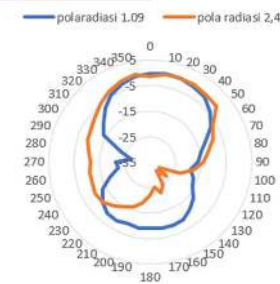
Gambar 30 Hasil Pengujian Pola Radiasi ADS-B dan S-Band
