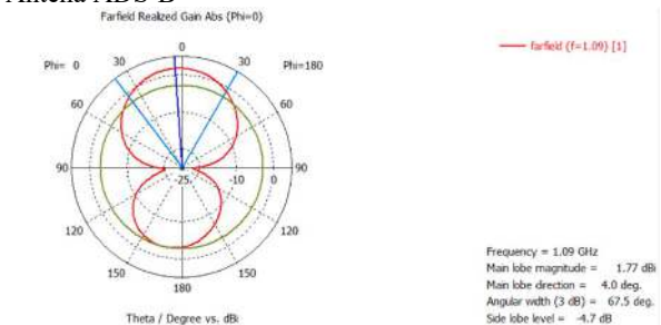
Gambar 22 Optimasi Gain dan Pola Radiasi ADS-B
