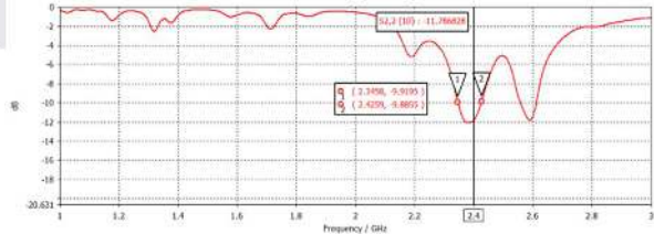
Gambar 19 Optimasi Return Loss S-Band
