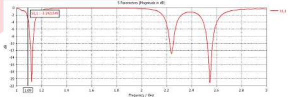
Gambar 10 Hasil Simulasi Pertama Return Loss ADS-B
