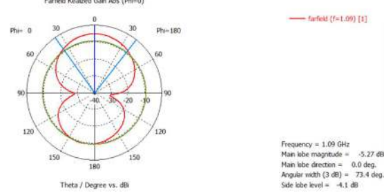
Gambar 14 Hasil Simulasi Pertama Gain ADS-B
