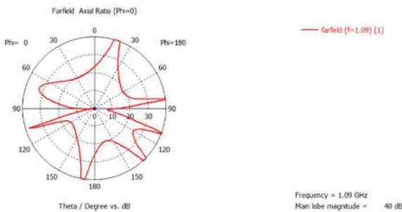
Gambar 24 Optimasi Polarisasi ADS-B
