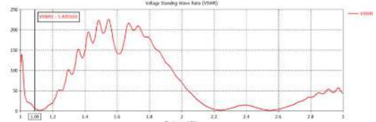
Gambar 12 Hasil Simulasi Pertama VSWR ADS-B
