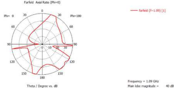
Gambar 16 Hasil Simulasi Pertama Polarisasi ADS-B
