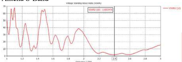
Gambar 21 Optimasi VSWR S-Band
