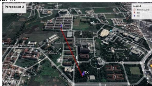
GAMBAR 8. Pengujian antar bagian kondisi 2
