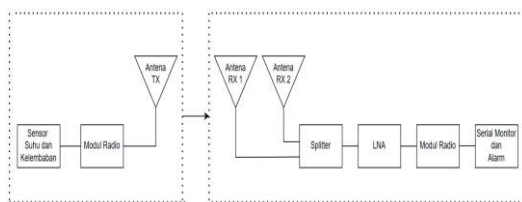
GAMBAR 2. Desain sistem keseluruhan
