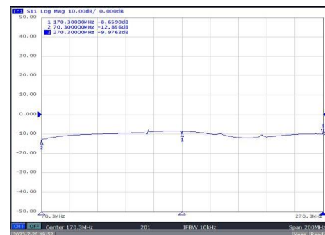
GAMBAR 4. Hasil pengukuran return loss
