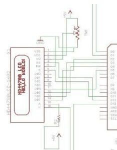
Gambar 3.5 Rangkaian LCD
