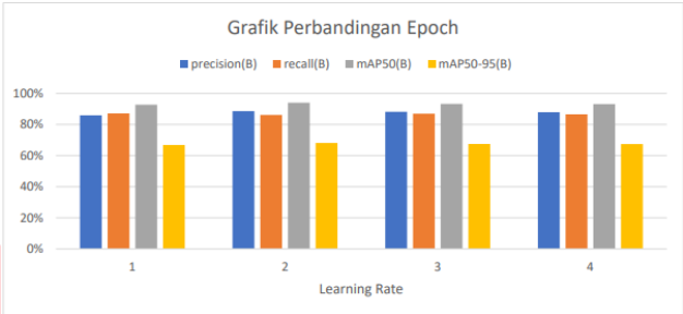
GAMBAR 13 pengujian epoch
