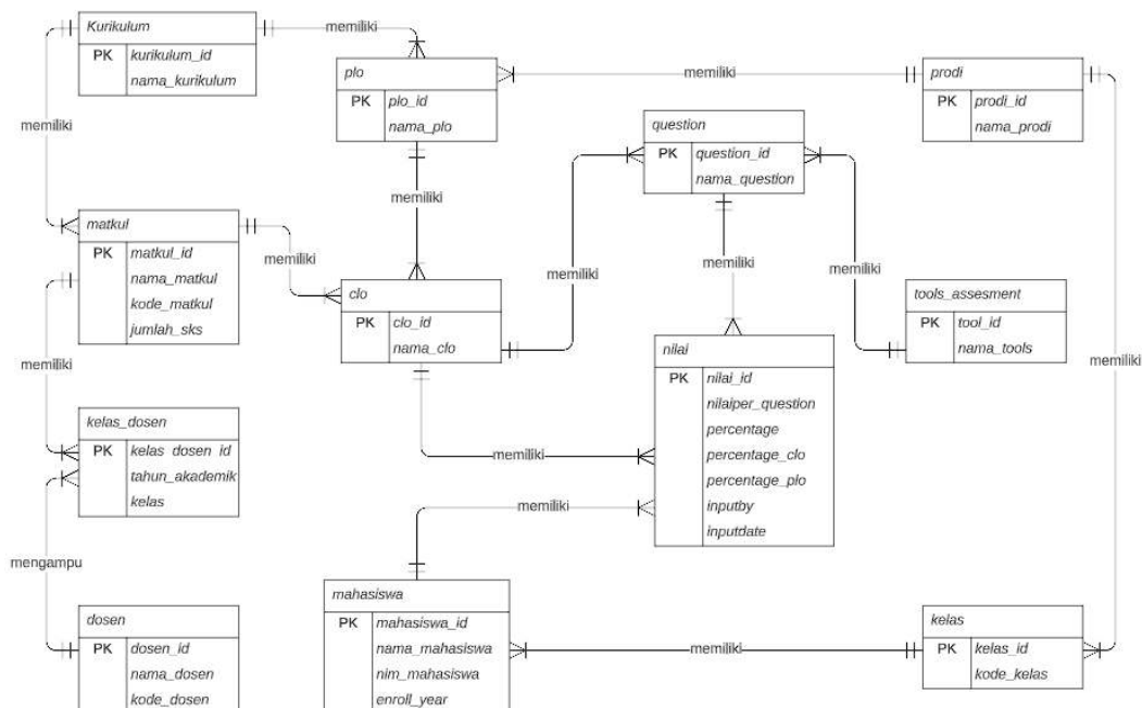
Gambar 3. 4 ERD akhir
