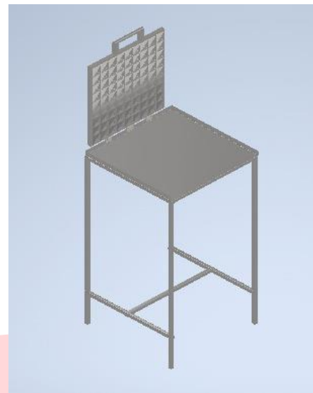
GAMBAR 9 Desain Rancangan Alat Bantu Potong
