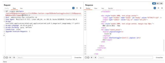
GAMBAR IV. 10 Output pengujian Kedua Menggunakan Burp Suite
