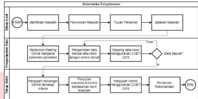
GAMBAR III. 2 Sistematika Penyelesaian Masalah
