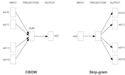
GAMBAR 4 Model CBOW dan Skip-Gram [28]
