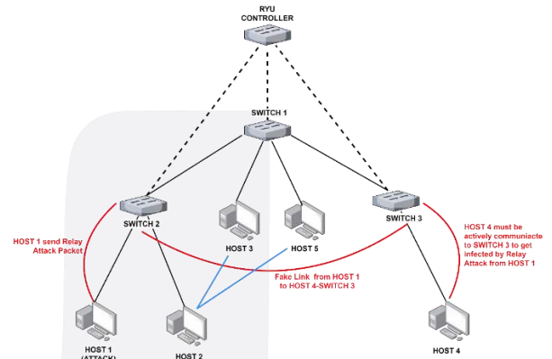
GAMBAR 1, TOPOLOGI JARINGAN(A)
