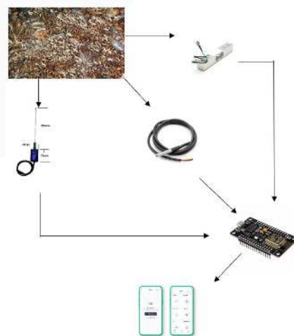
GAMBAR 7. Desain Perangkat Keras
