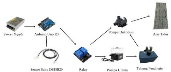
Gambar 3 Alur Keluar Masuk Air pada Pompa
