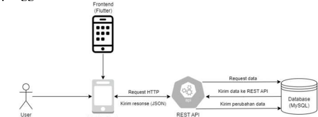
GAMBAR 3 (Rancangan Sistem Aplikasi)
