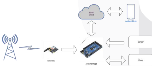
GAMBAR 1 Model Rancangan Sistem
