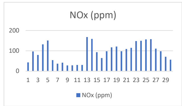
GAMBAR 5 Grafik NoX
