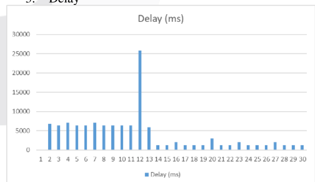
GAMBAR 7 Grafik Delay
