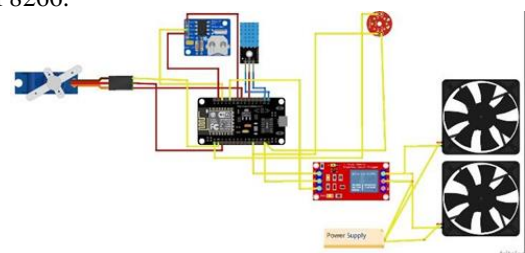
GAMBAR 4 (F) Rangkaian Skematik Sistem
