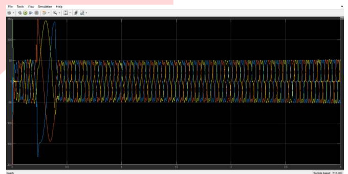
GAMBAR 8 Keluaran Iabc Sumber
