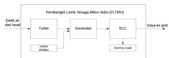
GAMBAR 1 Diagram Blok Simulasi PLTMH
