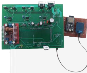
GAMBAR 4.1 Tampak Atas Sistem
