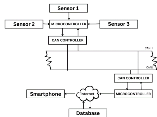
GAMBAR 3.1. Desain Sistem
