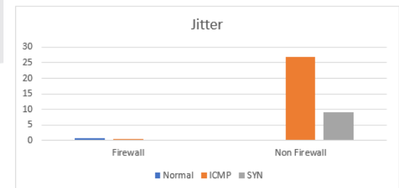
GAMBAR IV-7 Jitter
