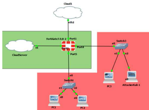
GAMBAR IV-1 Topologi
