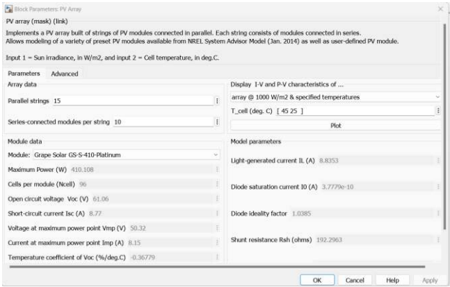
. GAMBAR 7 Parameter PV
