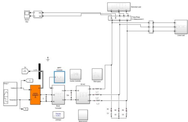
GAMBAR 6 Rangkaian PLTS
