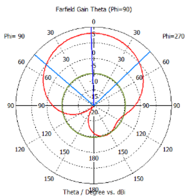
GAMBAR 3.5 Sudut Elevasi ( \Theta )
