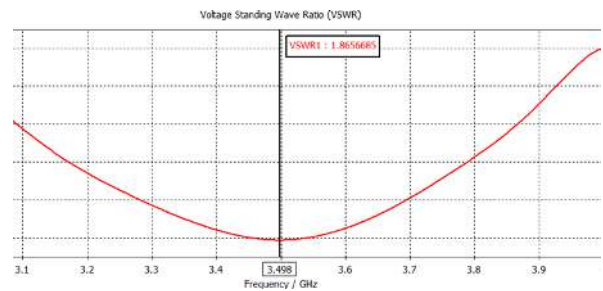
GAMBAR 3.7 Hasil simulasi nilai VSWR optimasi
