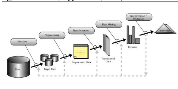
GAMBAR II-1 Tahapan KDD
