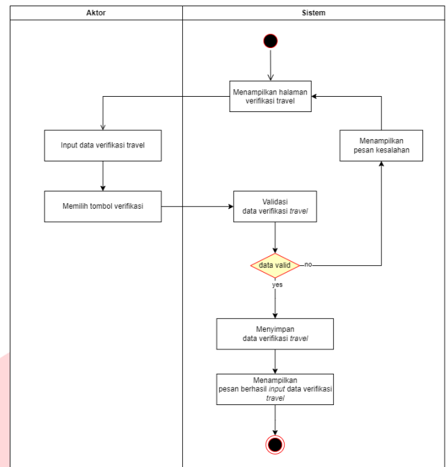
GAMBAR IV-3 Activity Diagram Create Konfirmasi Pendaftaran Travel Baru
