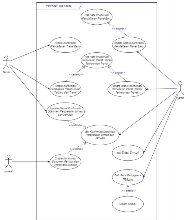
GAMBAR IV-1 Use Case Diagram Verifikasi
