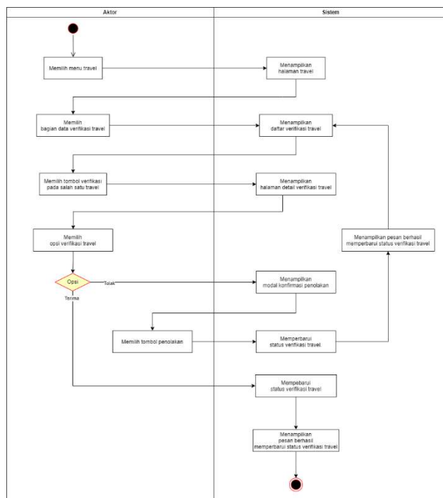
GAMBAR IV-2 Activity Diagram Update Status Konfirmasi Pendaftaran Travel Baru
