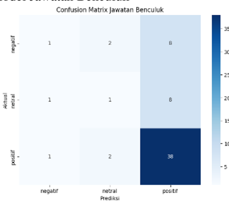
GAMBAR IV.4 (Confusion Matrix 3x3 Jawatan Benculuk)
