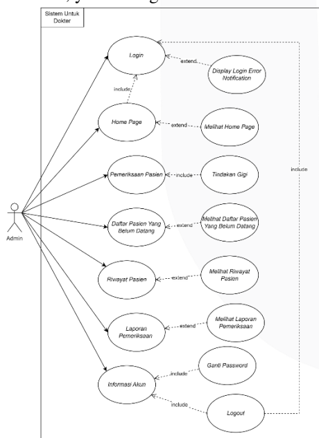
GAMBAR I. 10 Use Case Diagram Dokter
