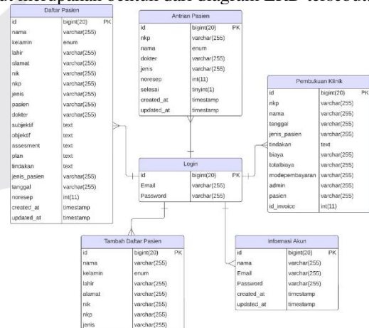
GAMBAR I. 8 Perancangan Entity Relationship Diagram (ERD)
