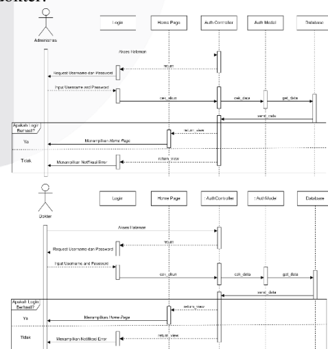
GAMBAR I. 12 Sequence Diagram Administrasi dan Dokter
