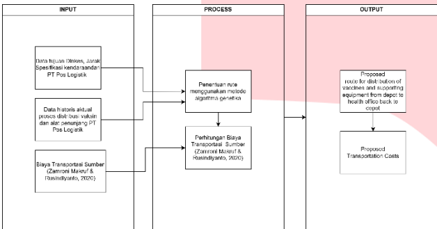
GAMBAR IV (Kerangka Berfikir)
