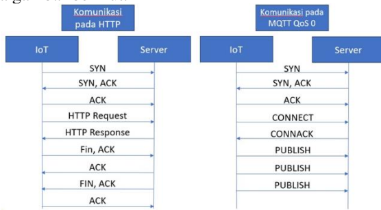
GAMBAR 4.4. Komunikasi pada HTTP dan MQTT
