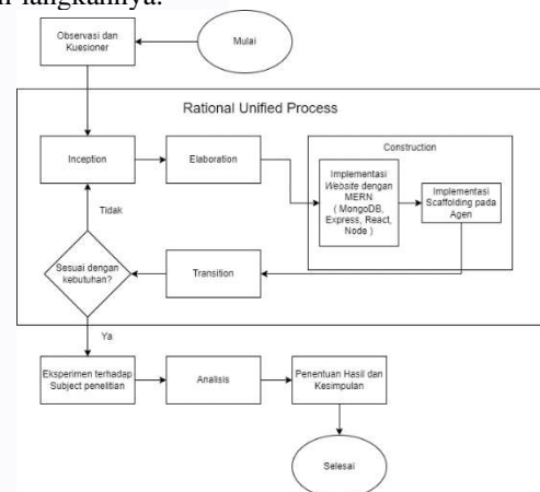
GAMBAR 2. Flowchart Aplikasi
