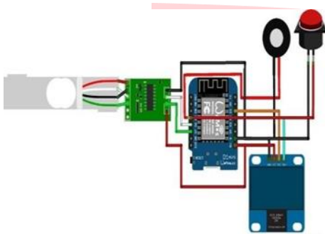
GAMBAR 5. Desain Perangkat Alat
