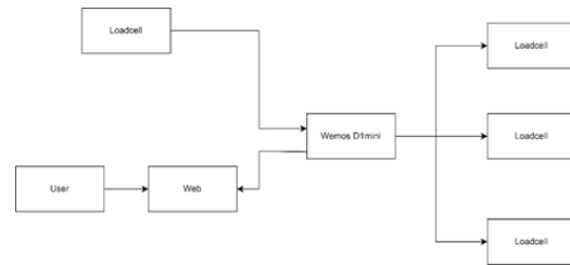
GAMBAR 3. Kalibrasi Komponen
