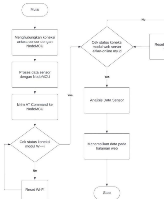
Gambar 3 Diagram Alir Kerja Alat
