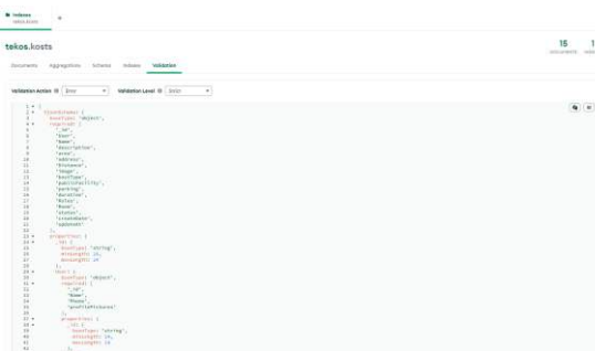
GAMBAR 3.3. Penerapan Pembatasan dan Validasi pada Tabel Kosti
