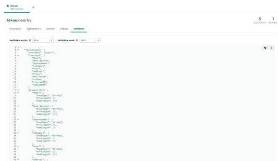
GAMBAR 3.5. Penerapan Pembatasan dan Validasi pada Tabel Nearby
