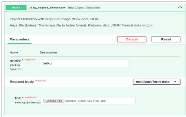
Fig. 4. JSON API Request
