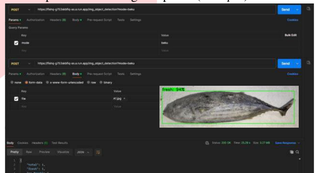
Fig. 6. Pengujian Ikan Cakalang Beku menggunakan aplikasi Postman
