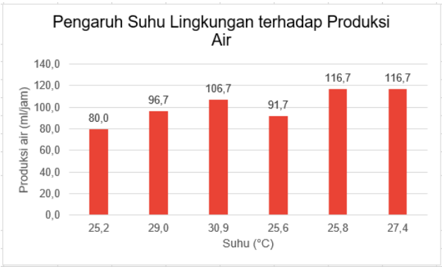
GAMBAR 4. Grafik pengaruh suhu lingkungan terhadap produksi air
