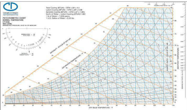
GAMBAR 2. Grafik Psikrometrik
